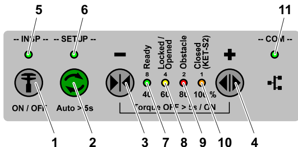
HMI Keypad [402032; 15.12.2014]
